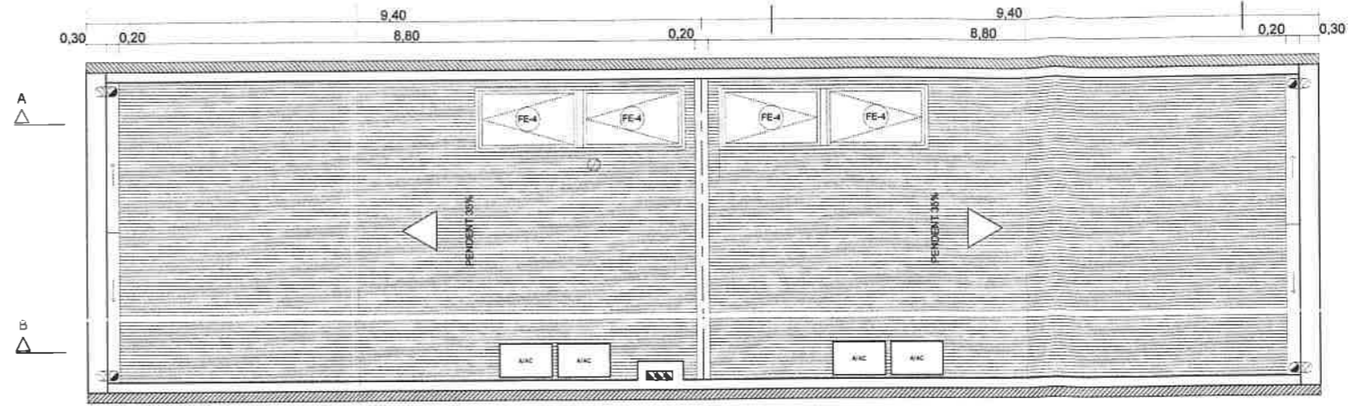
PLANTA COBERTA
