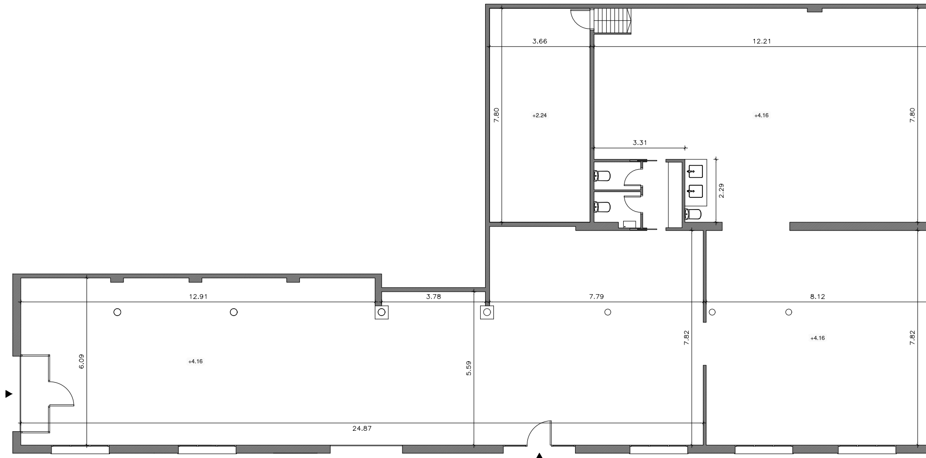
PLANTA LOCAL C/Loreto 37 Escala: 1/50
